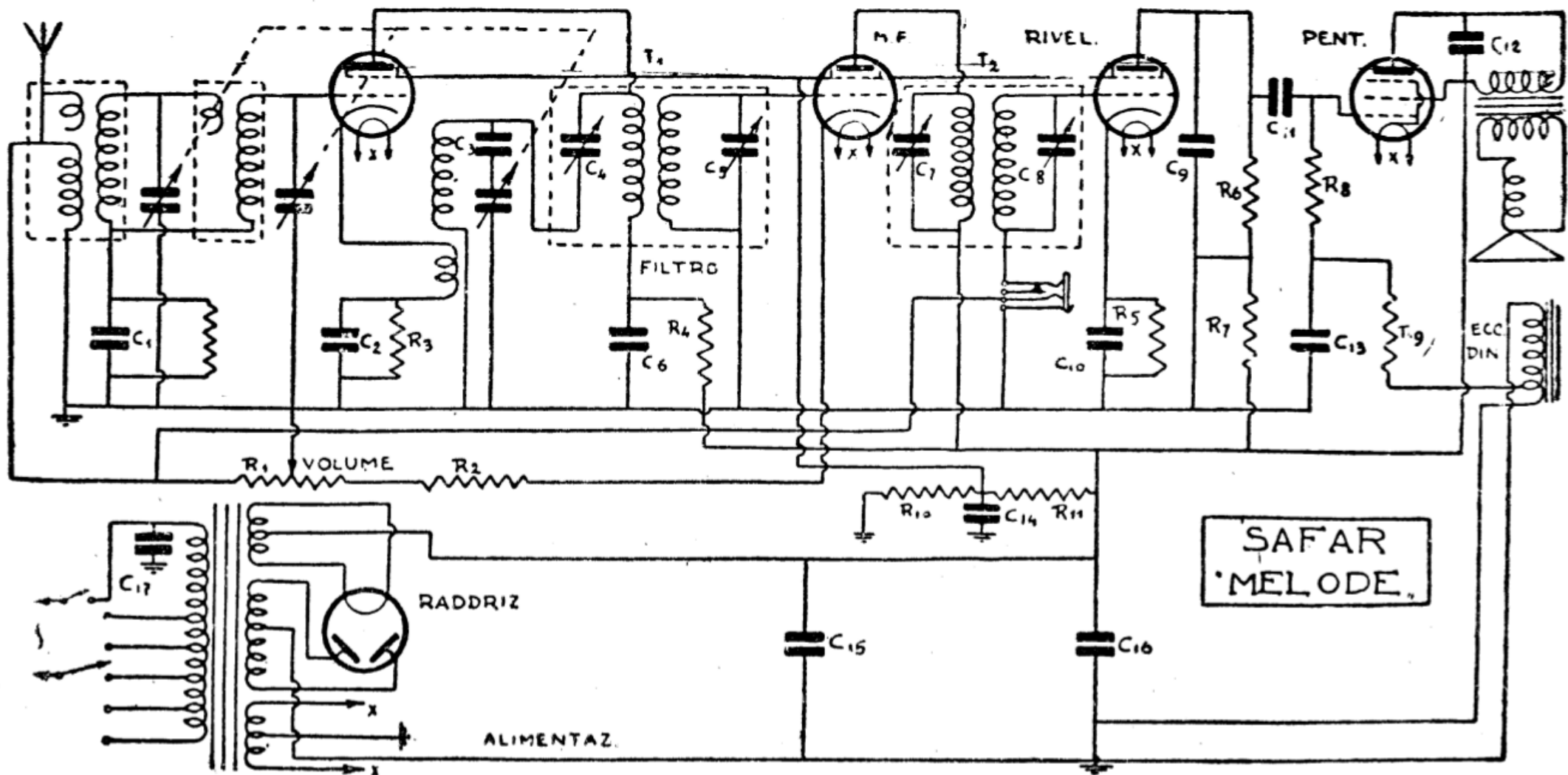
SAFAR RADIO. — Mod. Melode. — Valvole: V1 = '24; V2 = '35; V3 = '24; V4 = '47; V5 = '80. — MF: 175 kHz. Produzione 1932.
